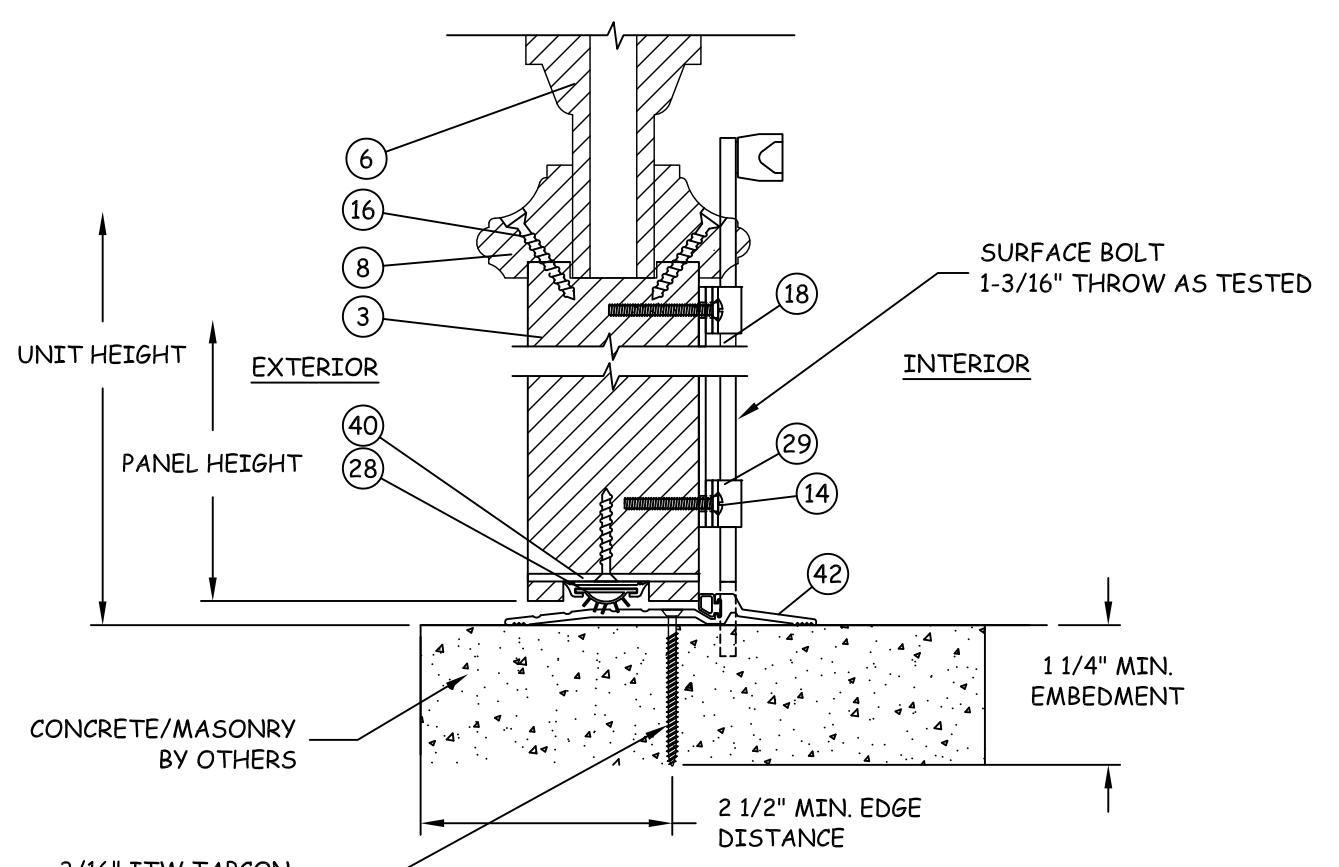
A2 9 VERTICAL SECTION DOOR SILL - CONCRETE/MASONRY ADA SILL
