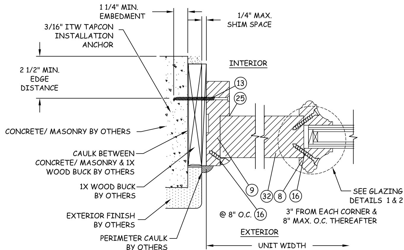
Q13 HORIZONTAL SECTION SIDELITE JAMB AT CONCRETE/MASONRY
